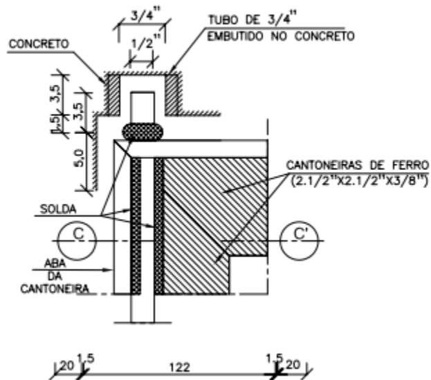
DETALHE DA ARTICULAÇÃO DA TAMPA ( VISTA INFERIOR )
